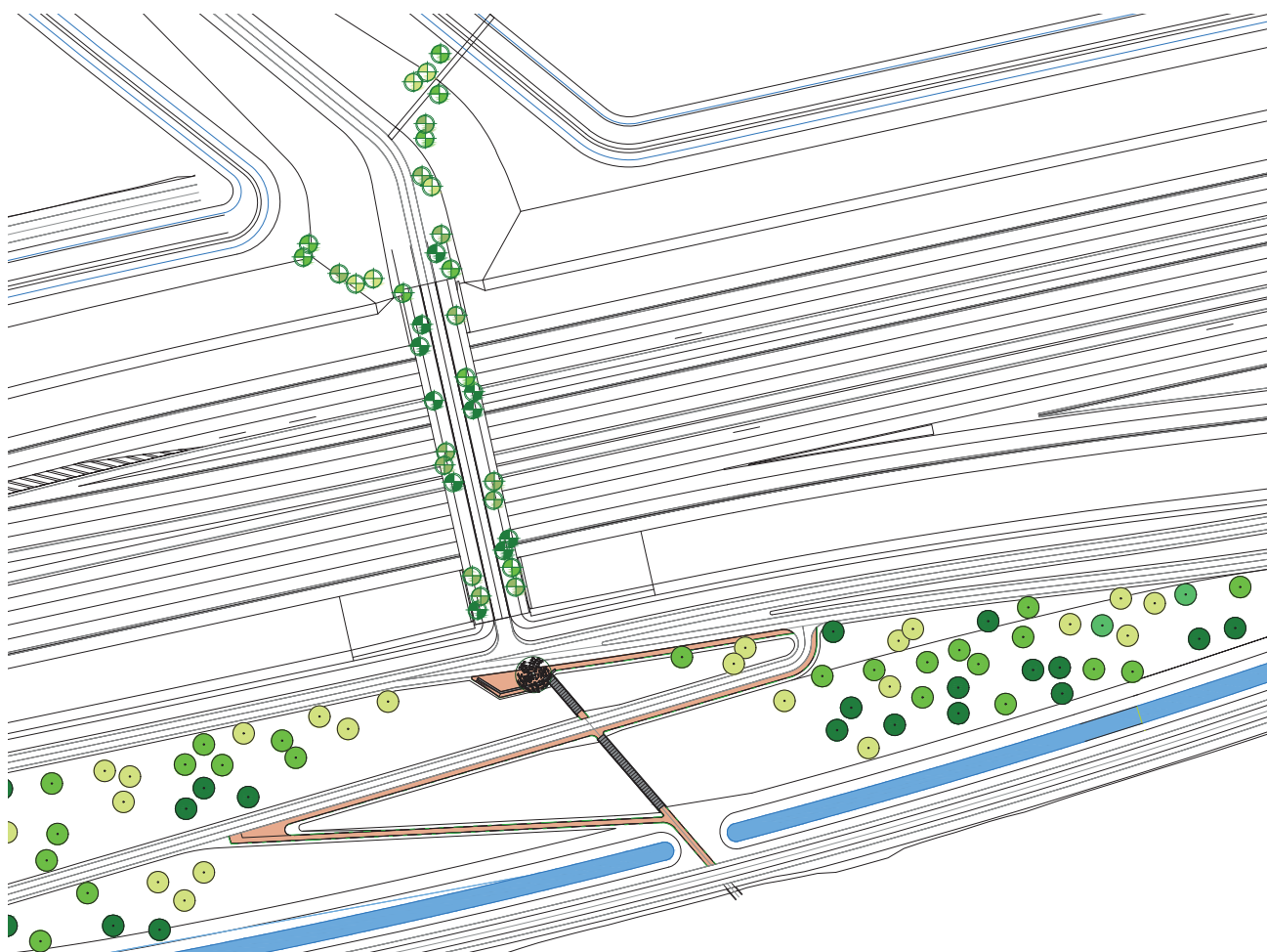
Recreaduct, aansluiting Schiebroeksepark, uitzichtpunt met zitplek
