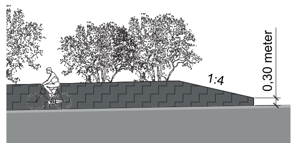
Uitwerking schanskorven, schuine beëindiging
