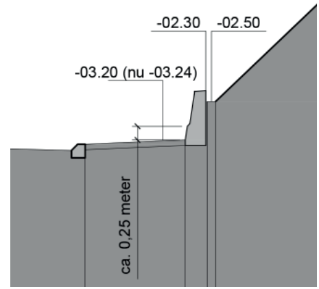
Doorsnede afwerking damplanken
