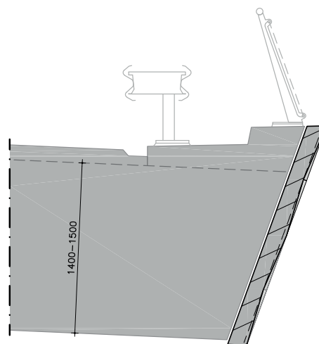
Randelementen viaducten
