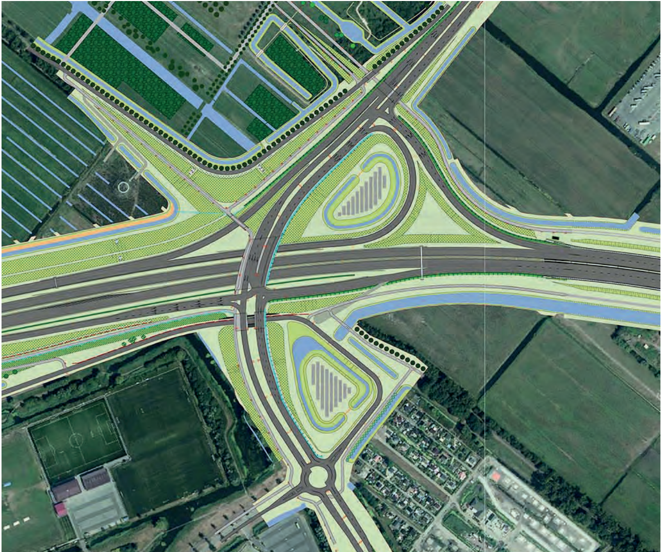
Landschappelijke inpassing Ankie Verbeek Ohrlaan (aansluiting Provinciale weg N209)
