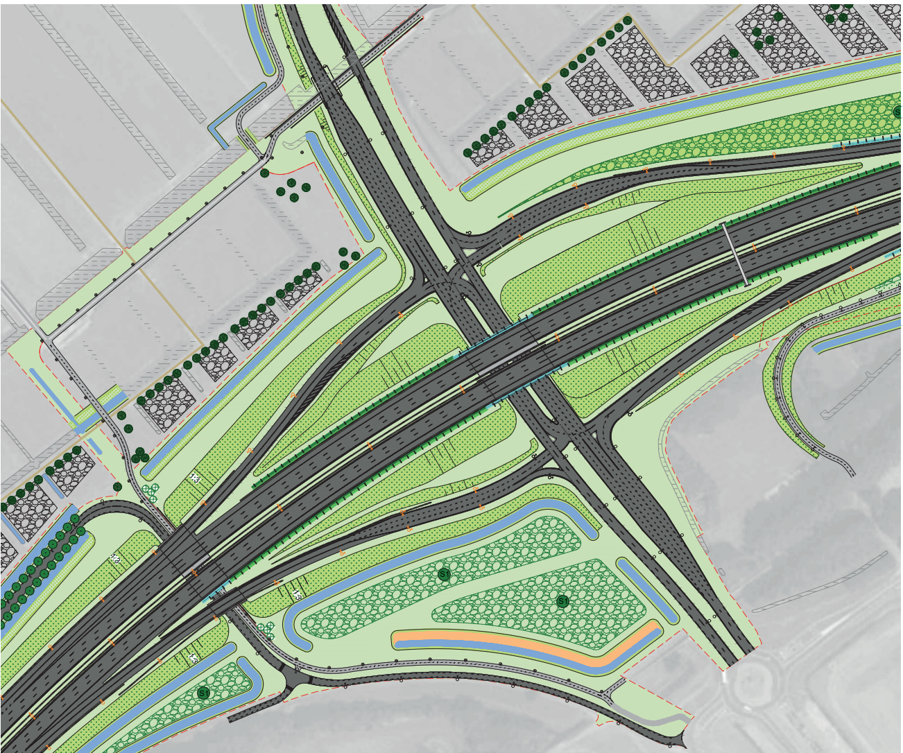
Landschappelijke inpassing Doenkadeviaduct (K20)
