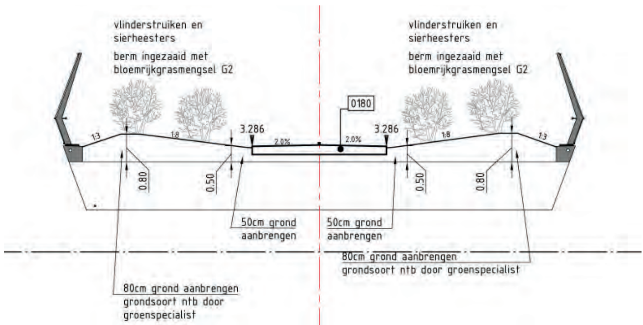
Doorsnede Recreaduct
