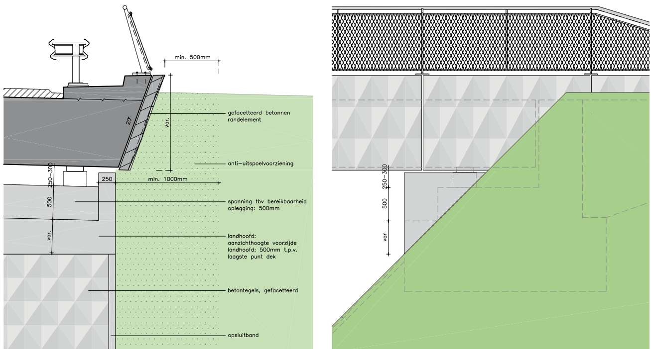
Detailering randelementen uit IPV
