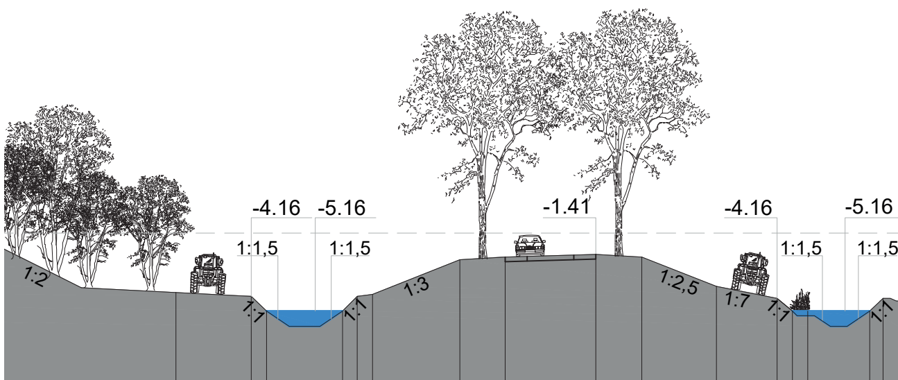
Doorsnede oprit naar vaste brug Schieveensedijk (K3)
