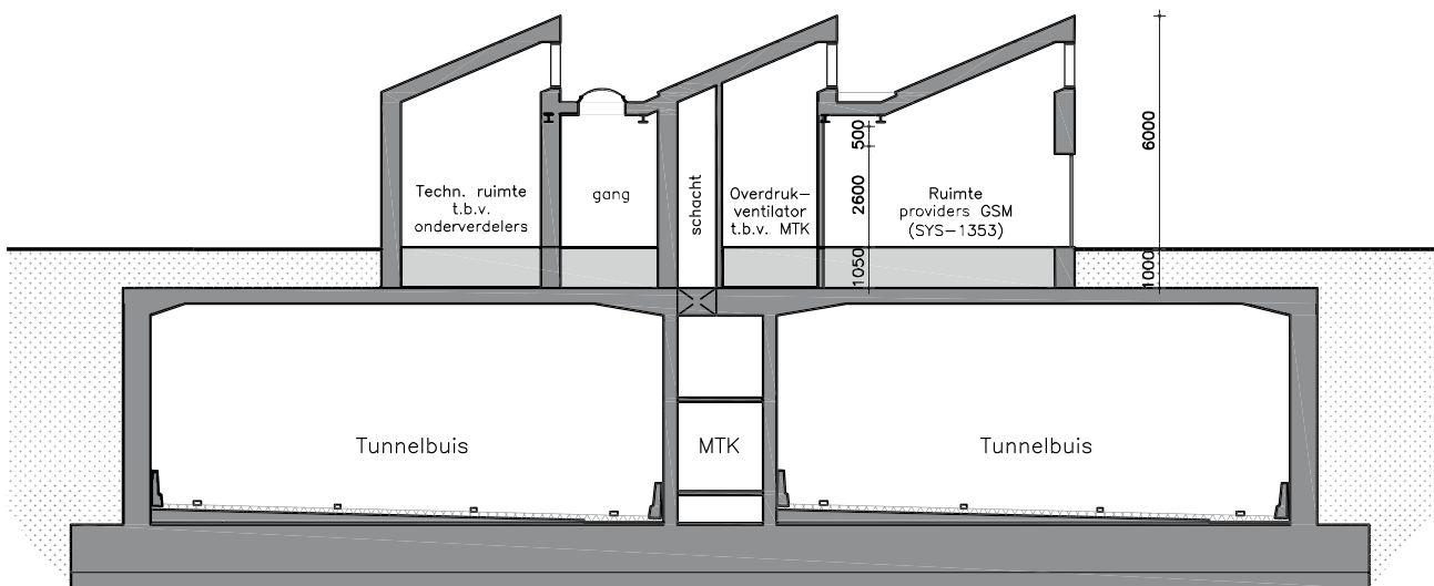
Doorsnede Dienstgebouw Zuid in relatie tot de tunnel
