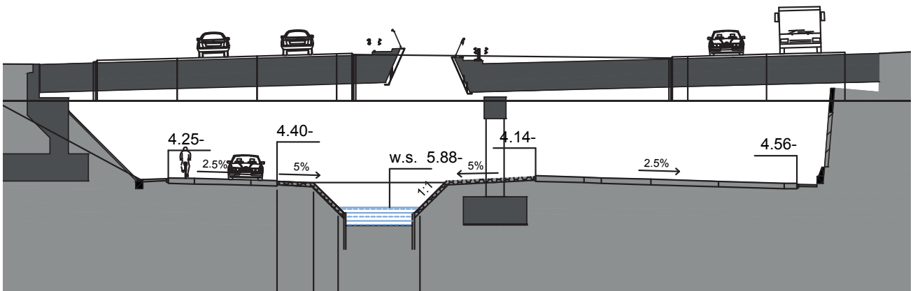
Doorsnede Viaduct Schieveensedijk (K10)
