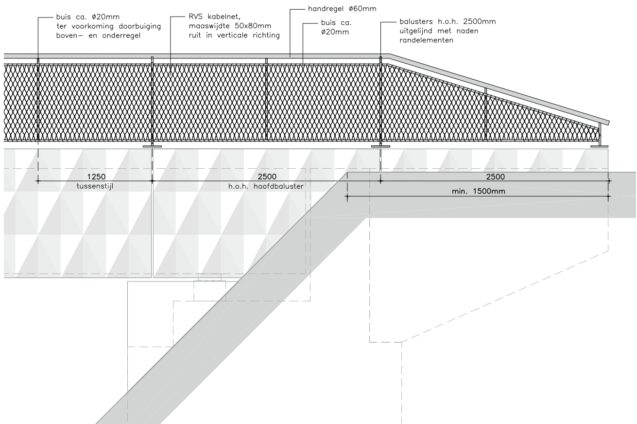
Detailering landhoofden en beëindiging randelementen
