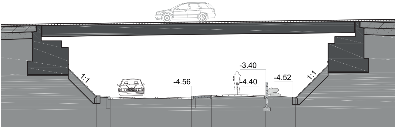
Doorsnede Tempelviaduct (K21) met rijweg, fietspad en faunapassage
