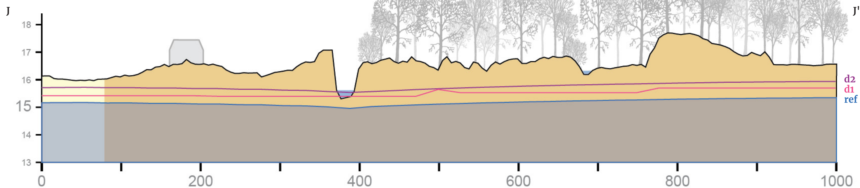
Fig. 123 Doorsnede J: zandruggen (centrale Achterhoek) met locatieaanduiding, indicatie van de GVG en grondwaterstandsverloop voor de huidige situatie (ref), denklijn 1 (d1) en denklijn 2 (d2)
