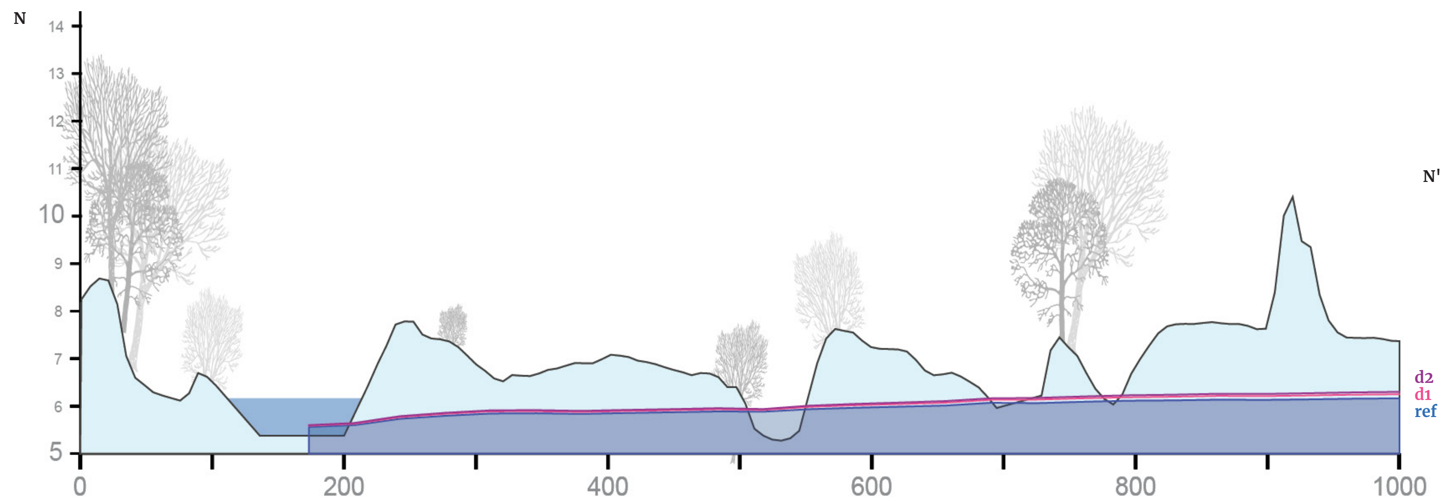
Fig. 127 Doorsnede N: grote rivieren met locatieaanduiding, indicatie van de GVG en grondwaterstandsverloop voor de huidige situatie (ref), denklijn 1 (d1) en denklijn 2 (d2)
