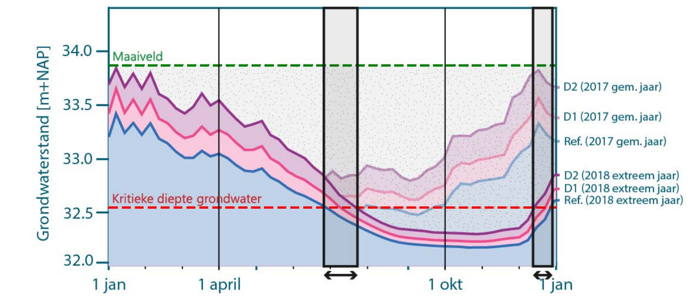
Tijdgrafiek grondwaterstanden (5)
