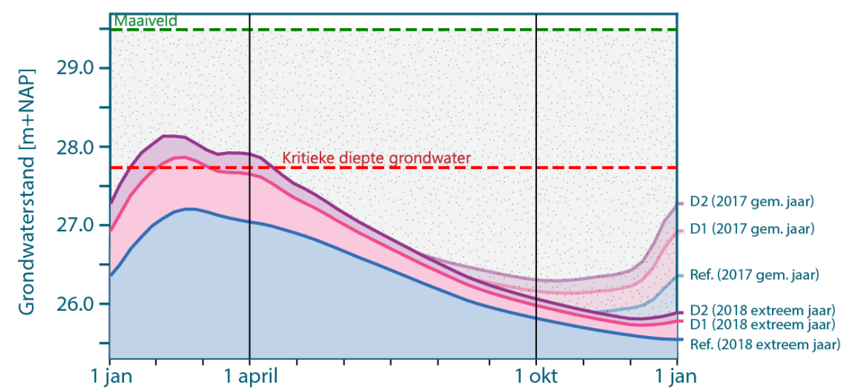
Tijdgrafiek grondwaterstanden (4)
