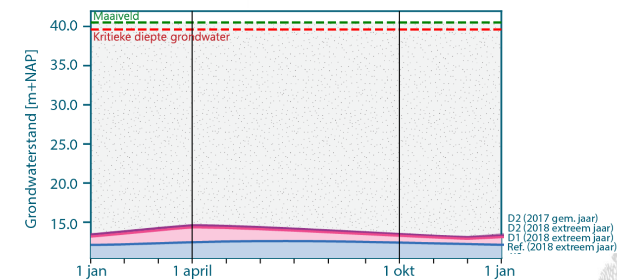
Tijdgrafiek grondwaterstanden (7)
