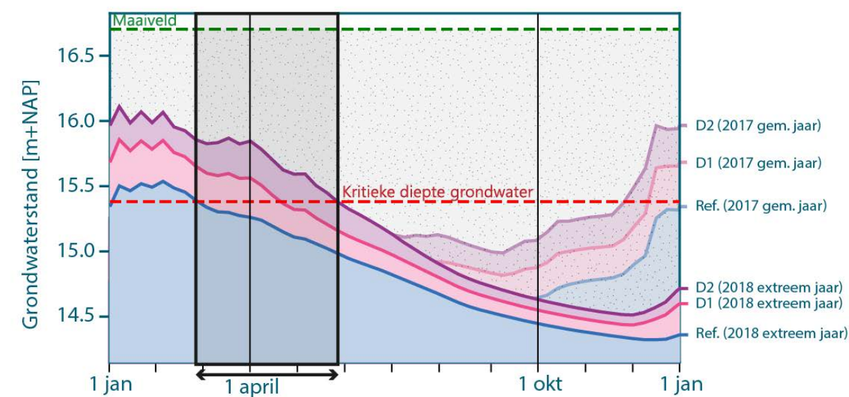
Tijdgrafiek grondwaterstanden (8)
