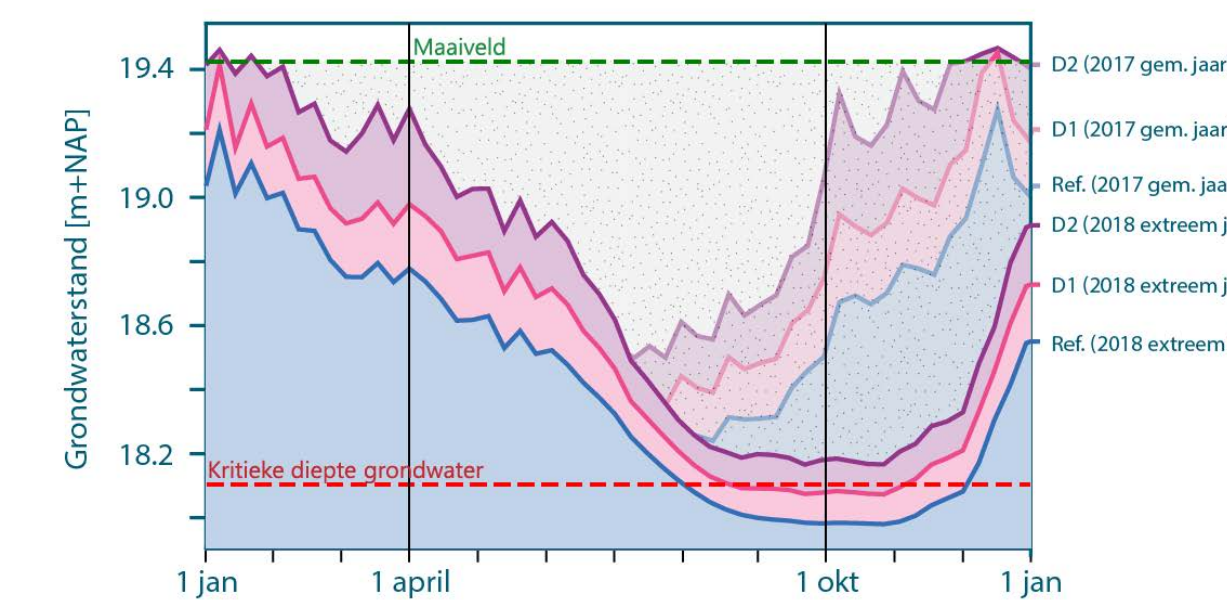
Tijdgrafiek grondwaterstanden (9)
