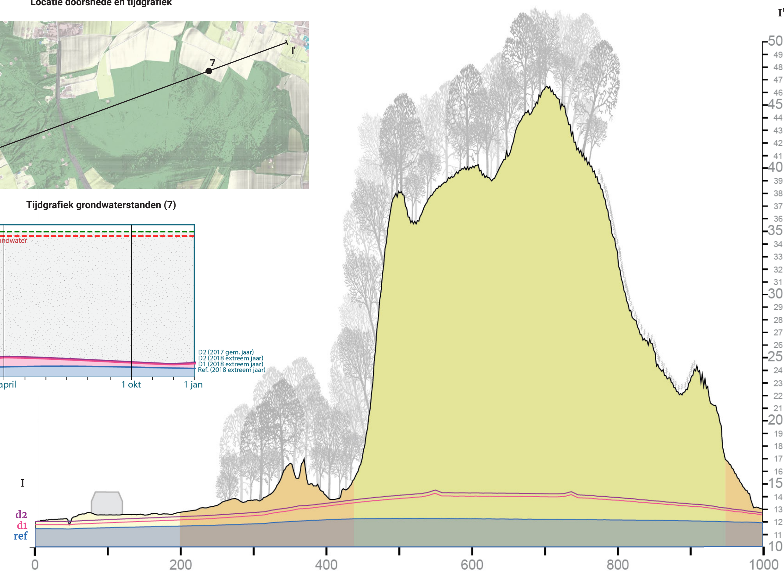
Fig. 122 Doorsnede I: stuwwal met locatieaanduiding, indicatie van de GVG en grondwaterstandsverloop voor de huidige situatie (ref), denklijn 1 (d1) en denklijn 2 (d2)
