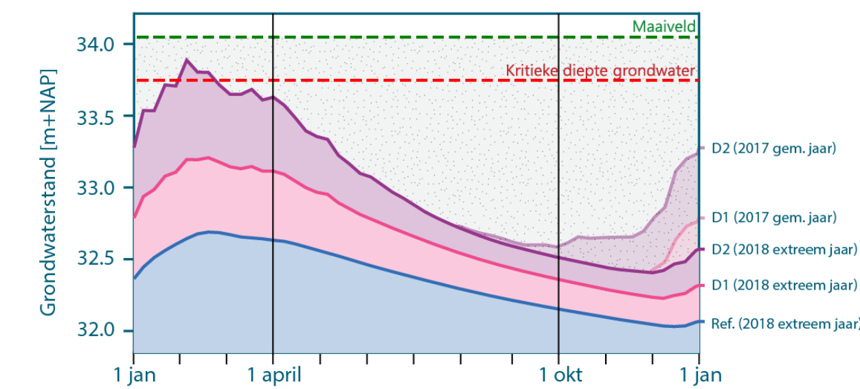
Tijdgrafiek grondwaterstanden (6)
