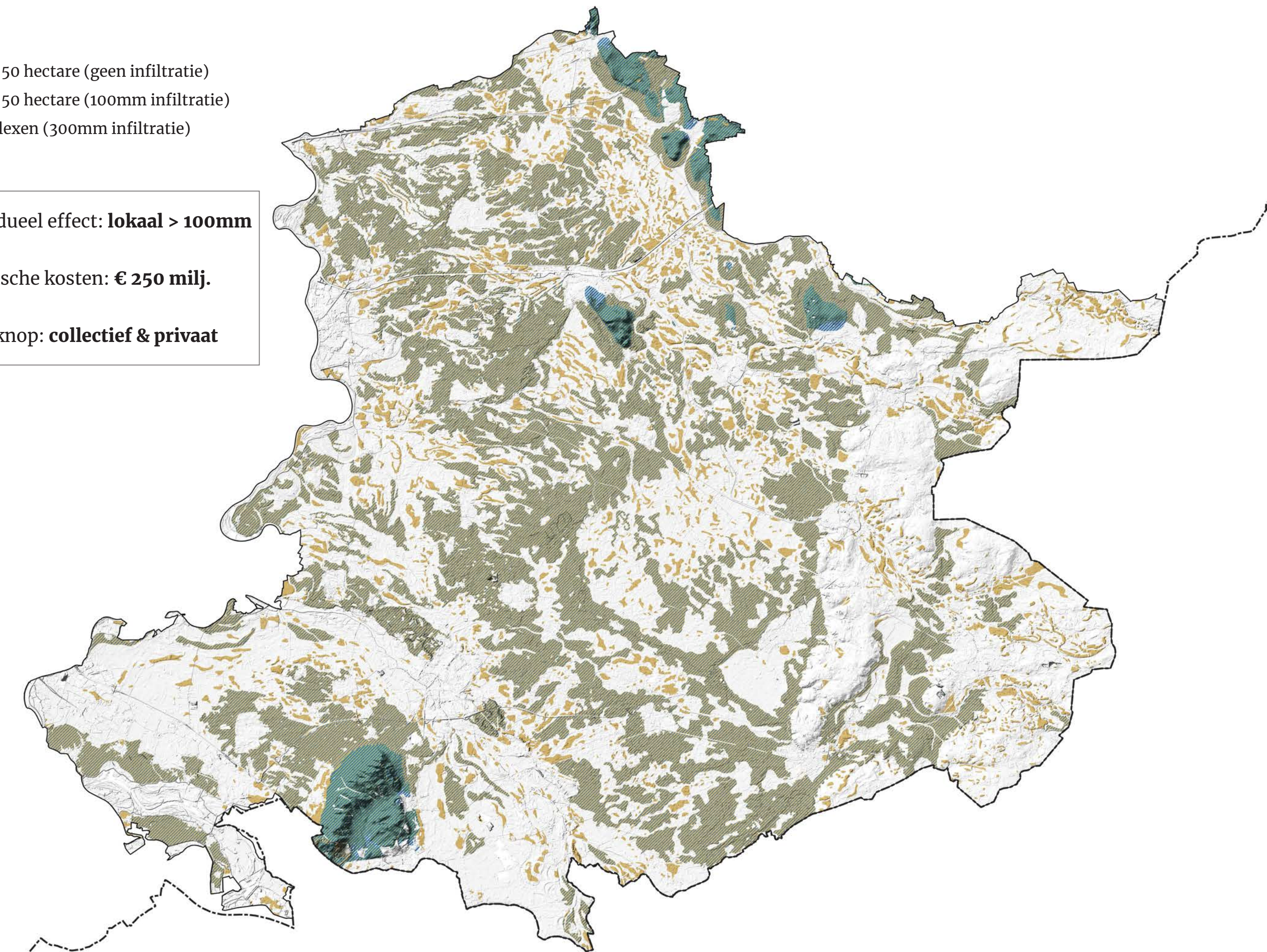
Fig. 106 Ligging zandruggen en stuwwalcomplexen >50 ha voor zoetwaterberging/infiltratie
