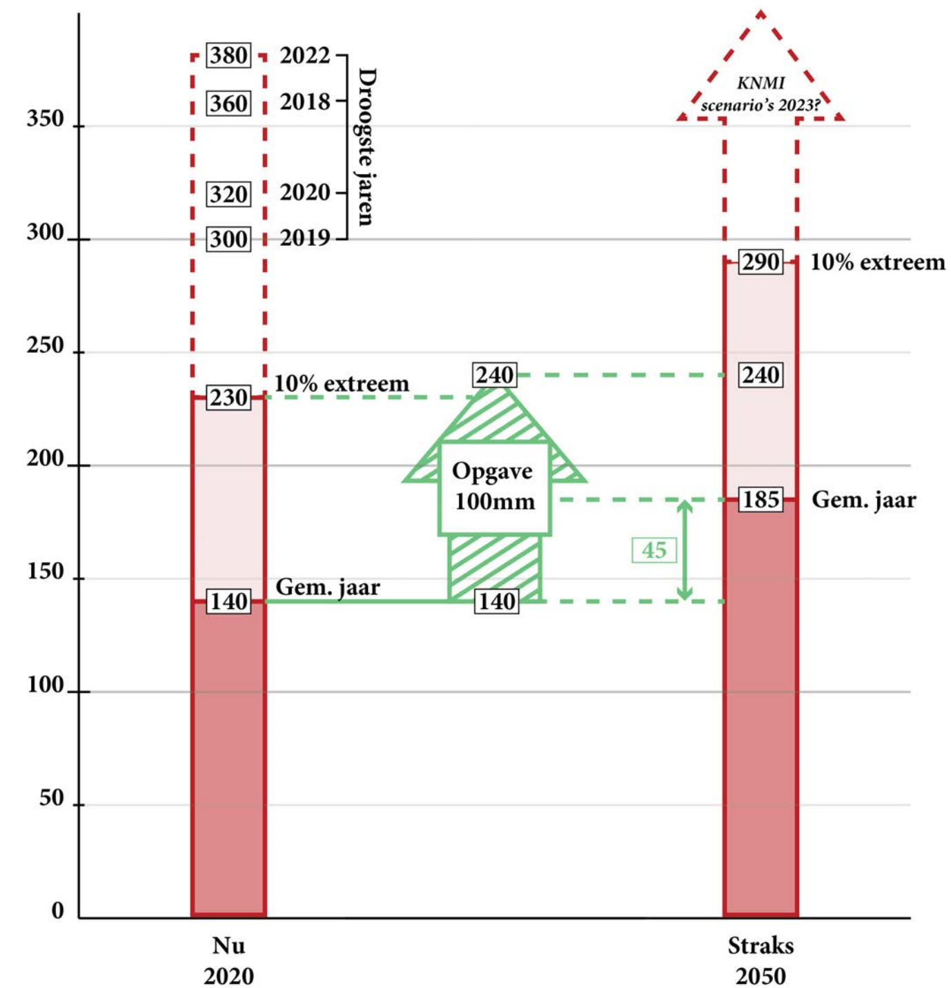
Fig. 24 Neerslagtekort in NL (gebaseerd op WH scenario's - KNMI, 2014)
